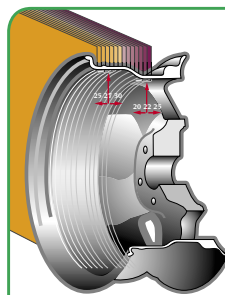
Programa Planos Móviles "Shift Plane" (en Alu P) para el uso de pesos múltiples de cinco gramos sin necesidad de efectuar cortes parciales (patente Corghi)
